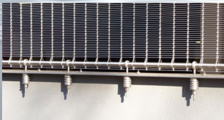
Untere Befestigung: Rundstange mit Augenschrauben und Druckfeder.
