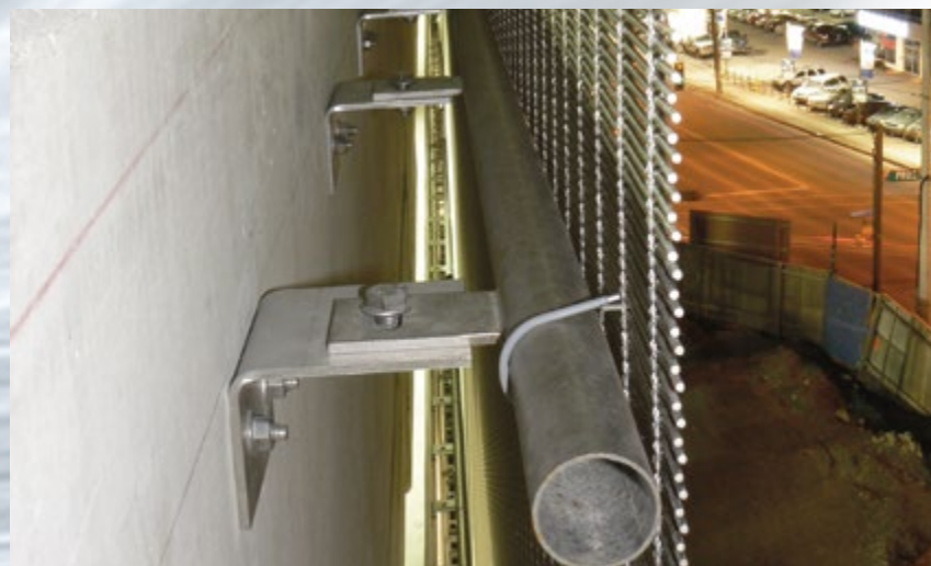
Zwischenbefestigung: Rundrohr und Drahtsicherung.
