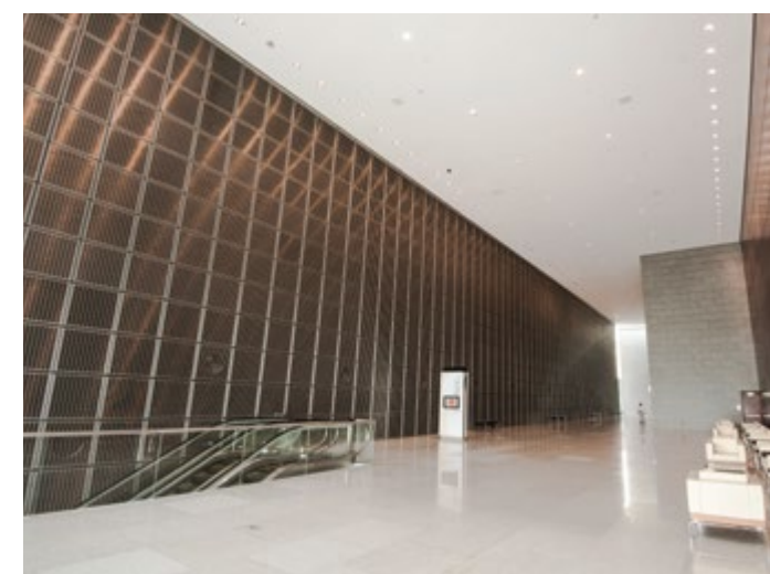
Gewebekassetten aus dem Architekturgewebe MULTI-BARRETTE 8123. Qatar National Convention Center, Doha, Katar.
