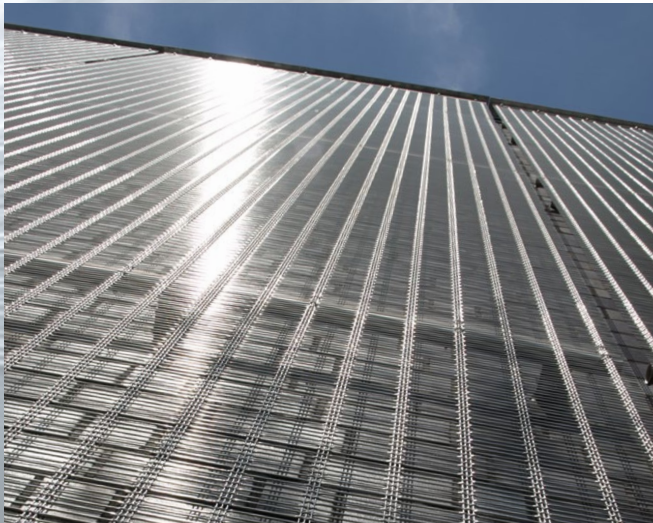
Architekturgewebe können über mehrere Geschosse hinweg vertikal gespannt werden. Tragende Unterkonstruktionen sind lediglich an der oberen und unteren Stirnseite erforderlich. Fassadenverkleidung DOGLA-TRIO 1032, Deutschland.
