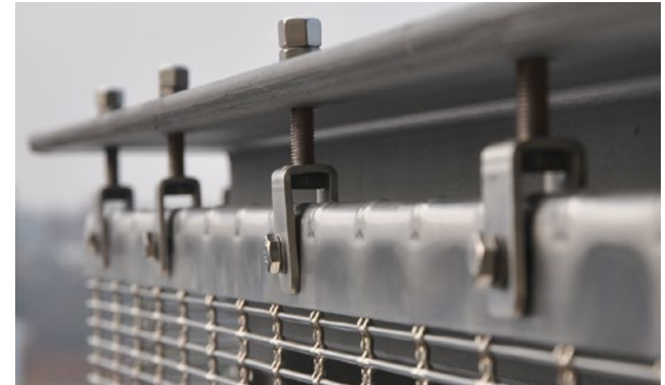
Obere Befestigung: Spannkante und Gabelschraube.
