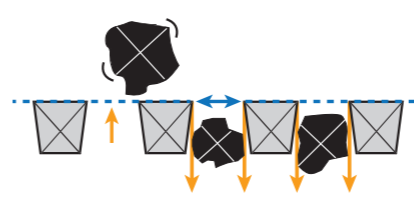
Des ouvertures coniques empêchent le colmatage. Le fond du tamis reste propre.
