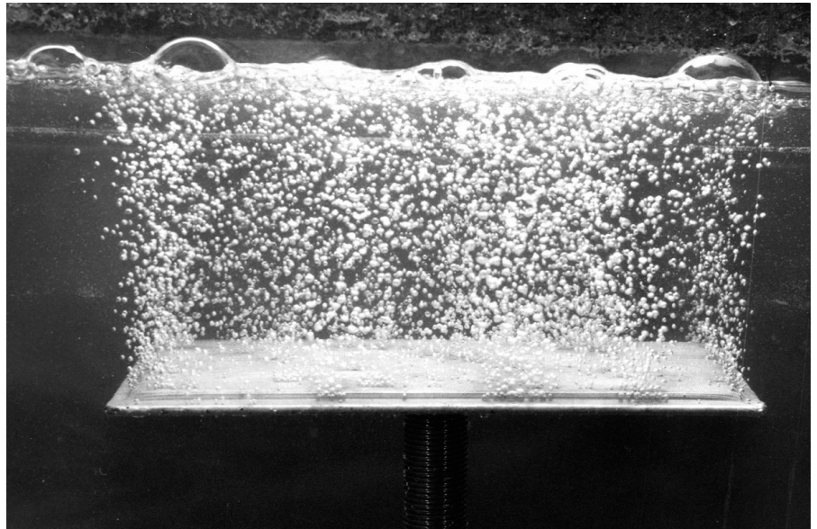
Gleichmäßige Durchströmung des PLYMESH-Belüftungskissens mit Luft, veranschaulicht im Wasserbad.
