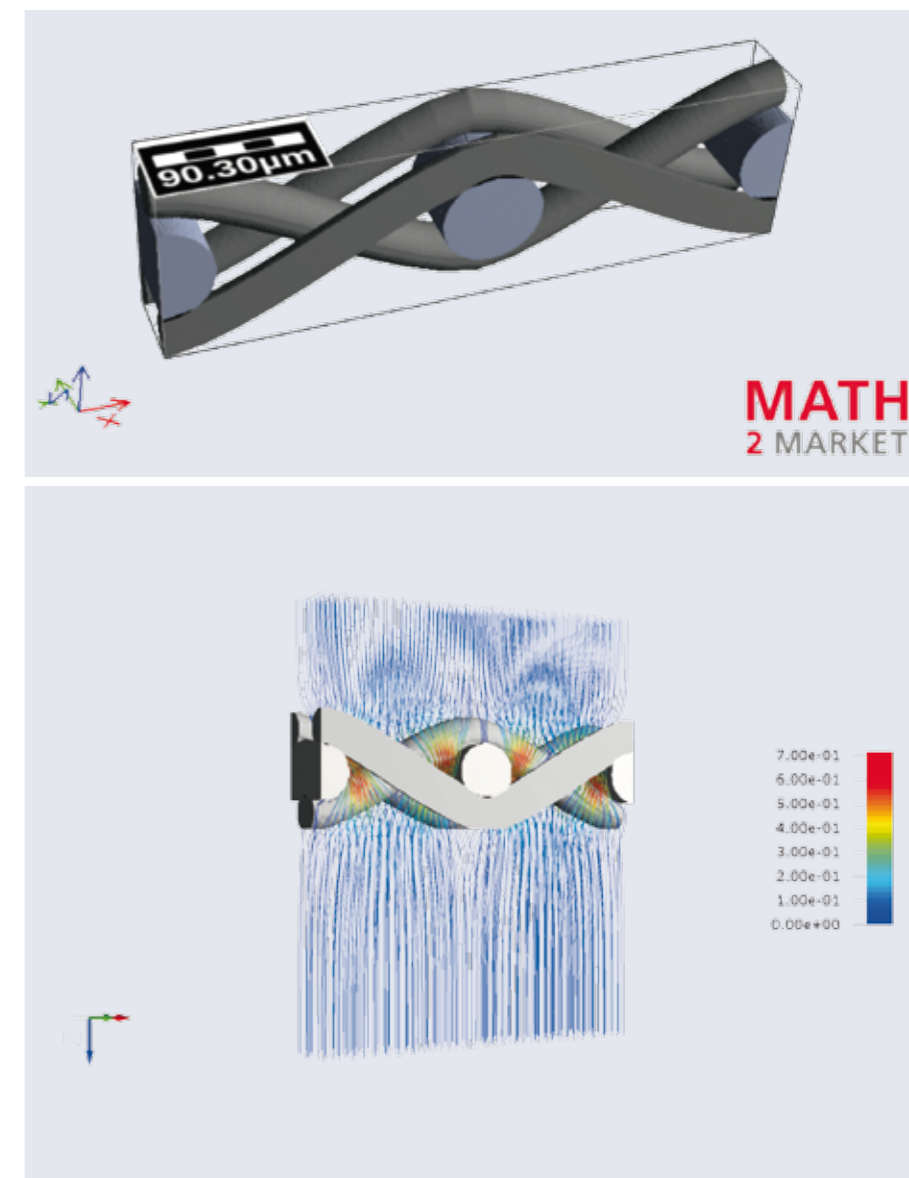
Die Gewebestruktur von MINIMESH® S-Filtertressen ist strömungsoptimiert.
