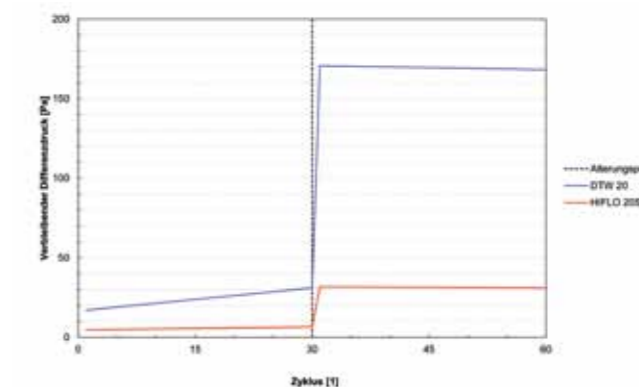
Abreinigungsverhalten in Anlehnung an VDI 3926
