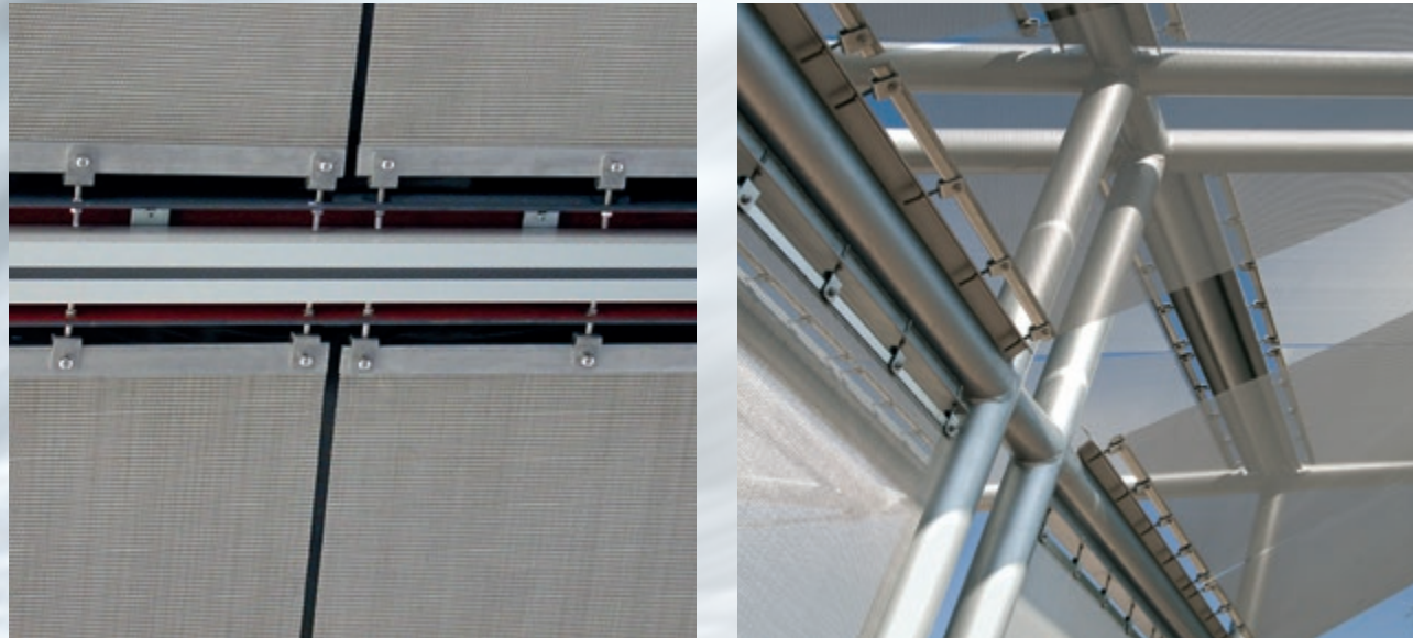
Système de fixation non modulaire pour plafonds avec profilé plat et vis à œillet.
