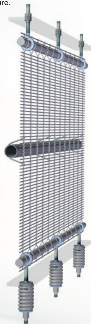
Technique de fixation pour façades en toile à mailles câblées.
