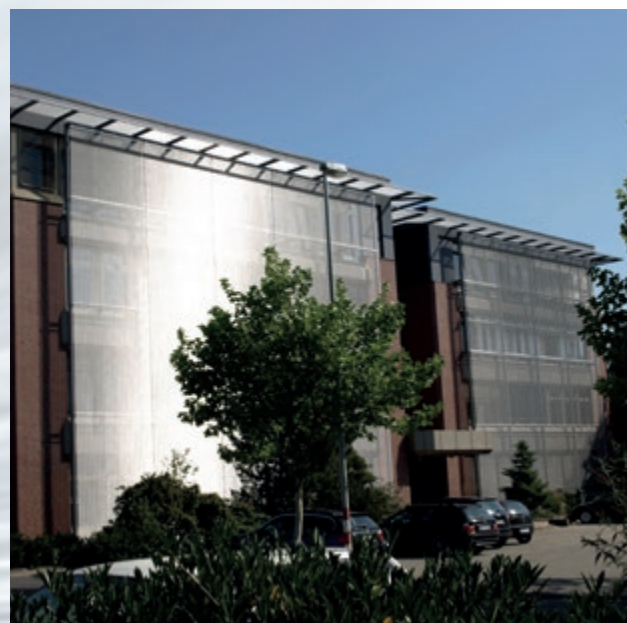
La maille métallique DOGLA-TRIO 1030 relie d'un point de vue visuel le nouvel étage surélevé à l'ancien bâtiment. Haver & Boecker, Oelde, Allemagne.
