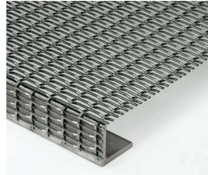
Maille métallique replié à 90° et soudé sur un profilé en L.
